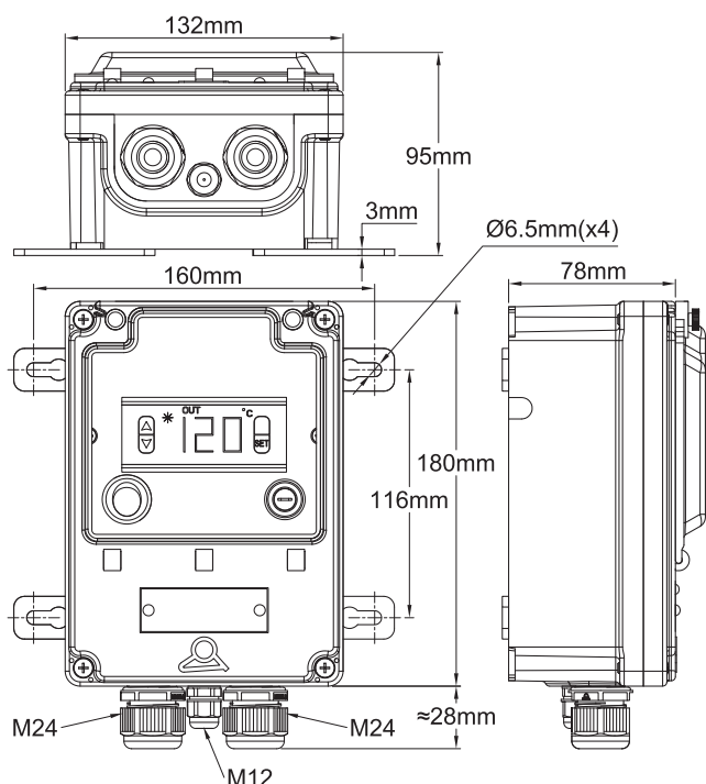
带 3 个电缆接头的型号 (2 × M24+1 × M12): Y8WH-X
