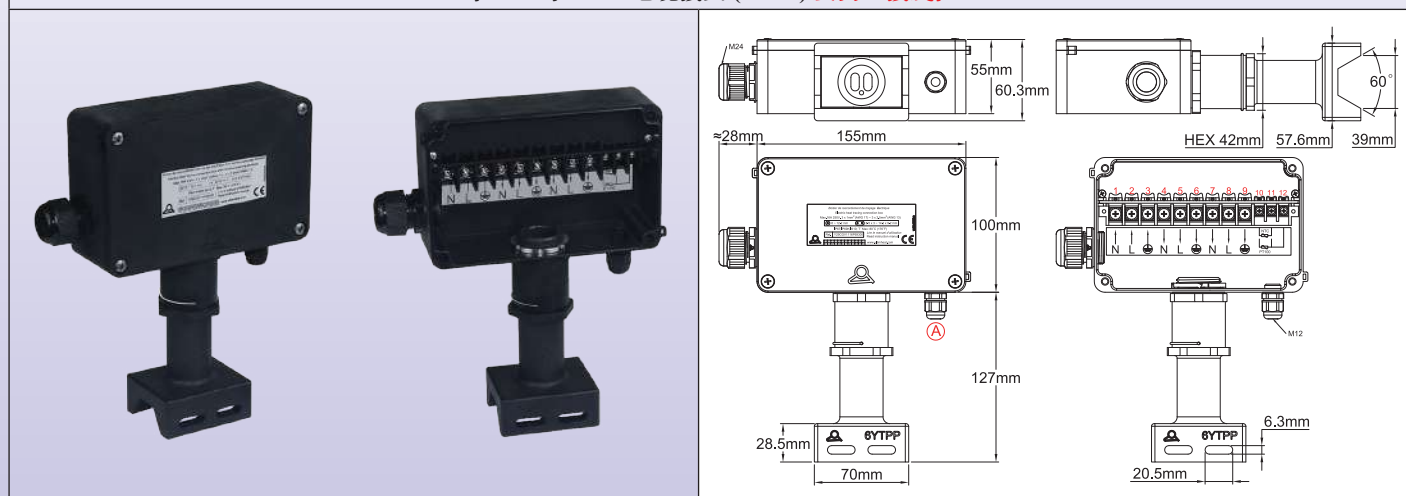
带 M24 和 M12 电缆接头 (Y29C) 及用于客户的接线柱的导轨
