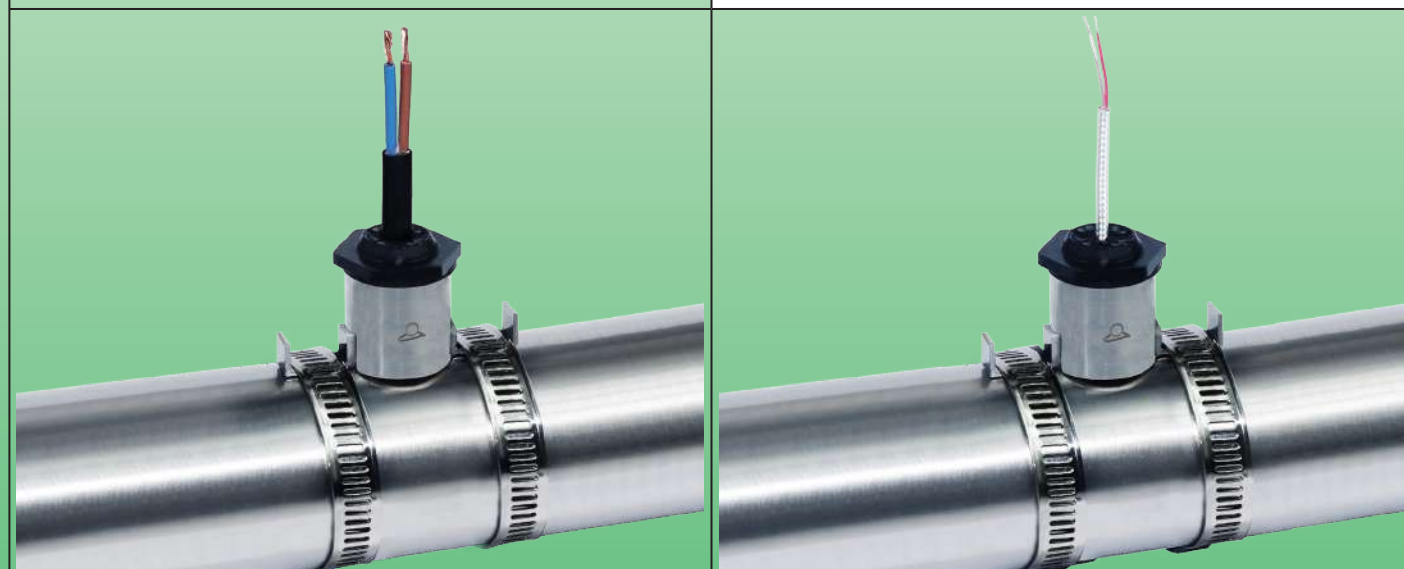
碟型温控器型号 49JB 安装在管道上的示例
