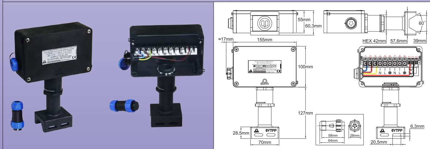
带 5 位连接器 (Y29D)
